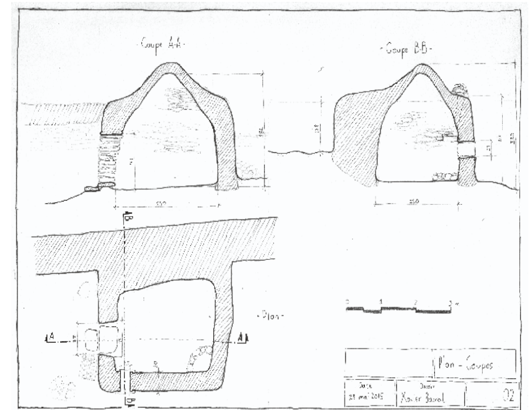
Plan coupe
